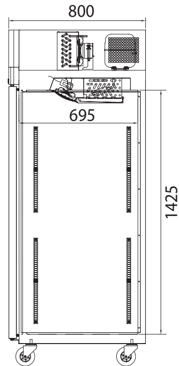
ВИД СБОКУ
