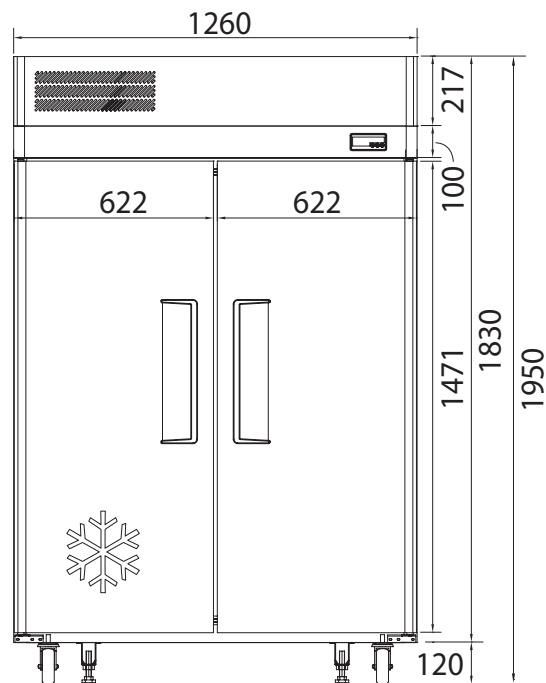
ВИД СПЕРЕДИ
