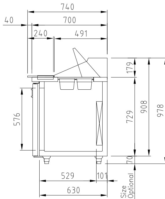
ВИД СБОКУ
