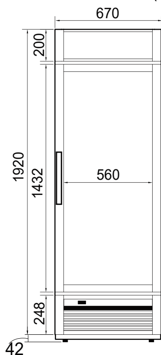
ВИД СПЕРЕДИ
