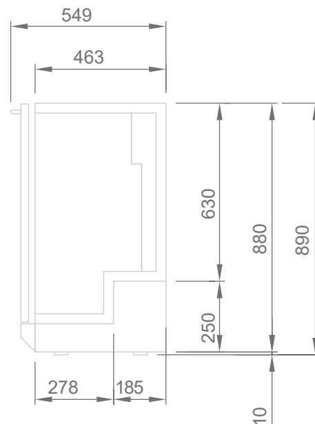
ВИД СБОКУ
