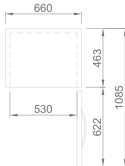
ВИД СВЕРХУ
