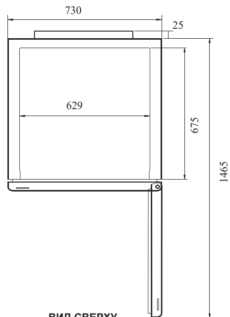
ВИД СВЕРХУ
