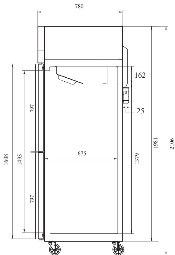
ВИД СБОКУ
