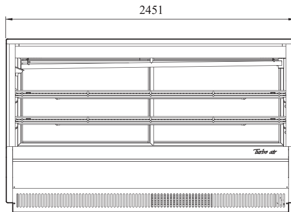
ВИД СПЕРЕДИ
