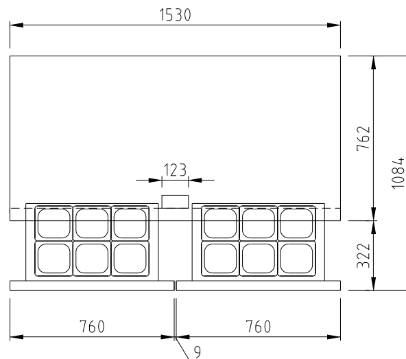
ВИД СВЕРХУ
