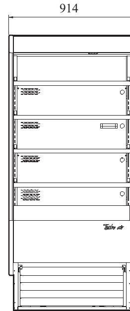
ВИД СПЕРЕДИ
