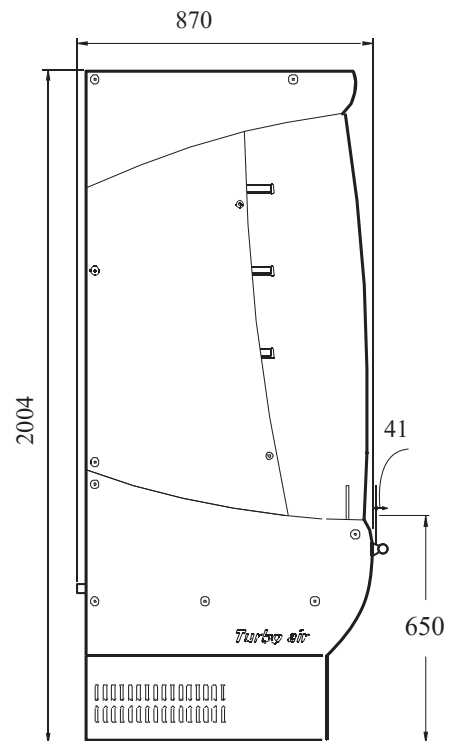
ВИД СБОКУ
