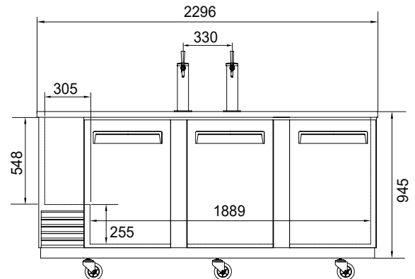
ВИД СПЕРЕДИ
