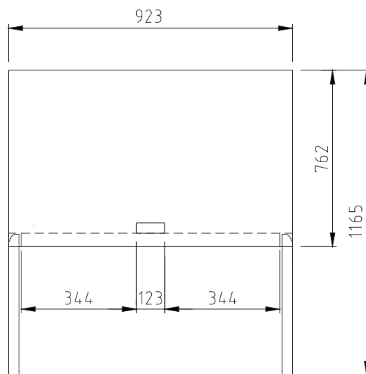
ВИД СВЕРХУ
