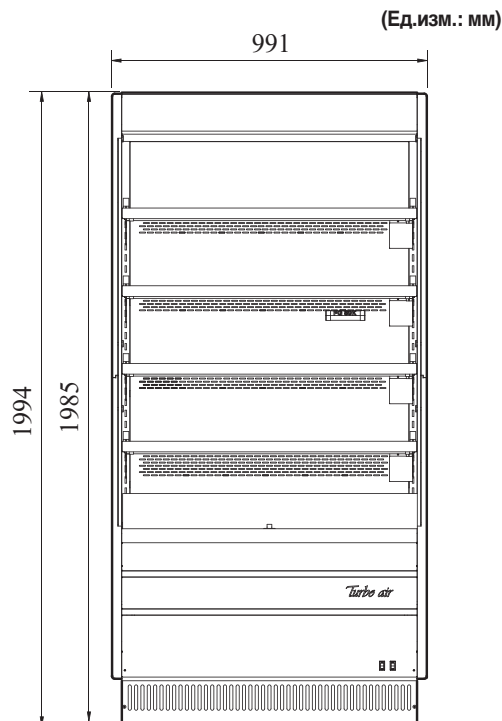
ВИД СПЕРЕДИ
