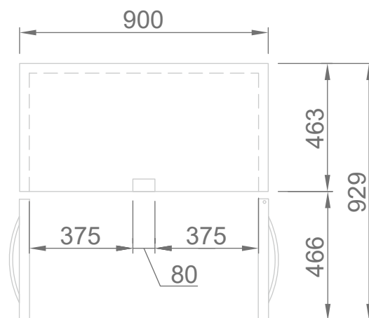
ВИД СВЕРХУ
