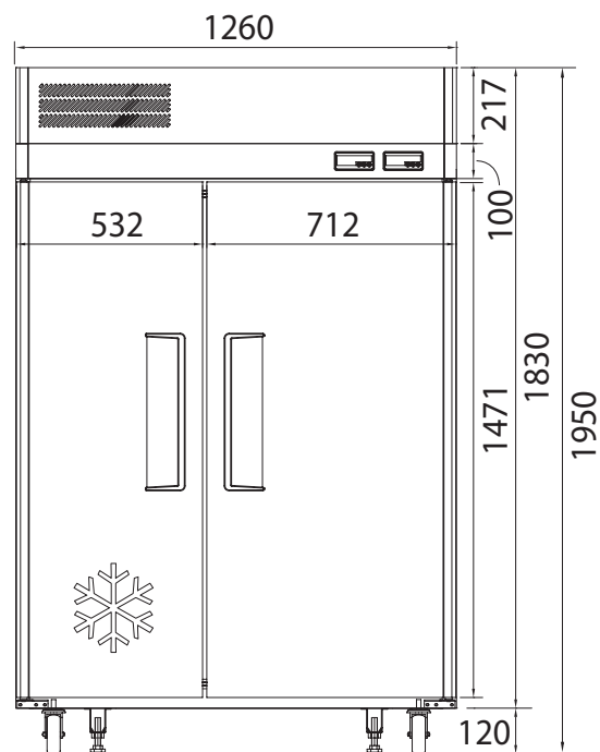
ВИД СПЕРЕДИ
