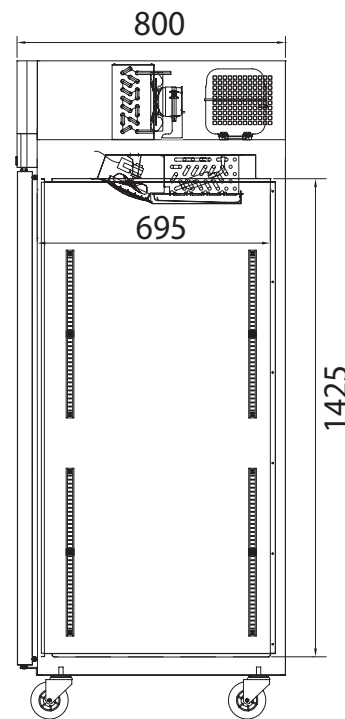
ВИД СБОКУ
